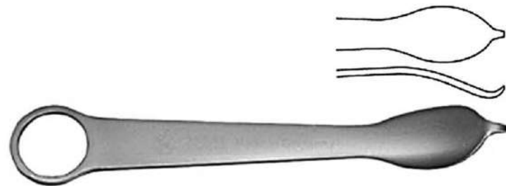
MI-11-01-0489 Hohman, Mini Bone Lever 12 cm / 4 3/4" 14 mm tip
